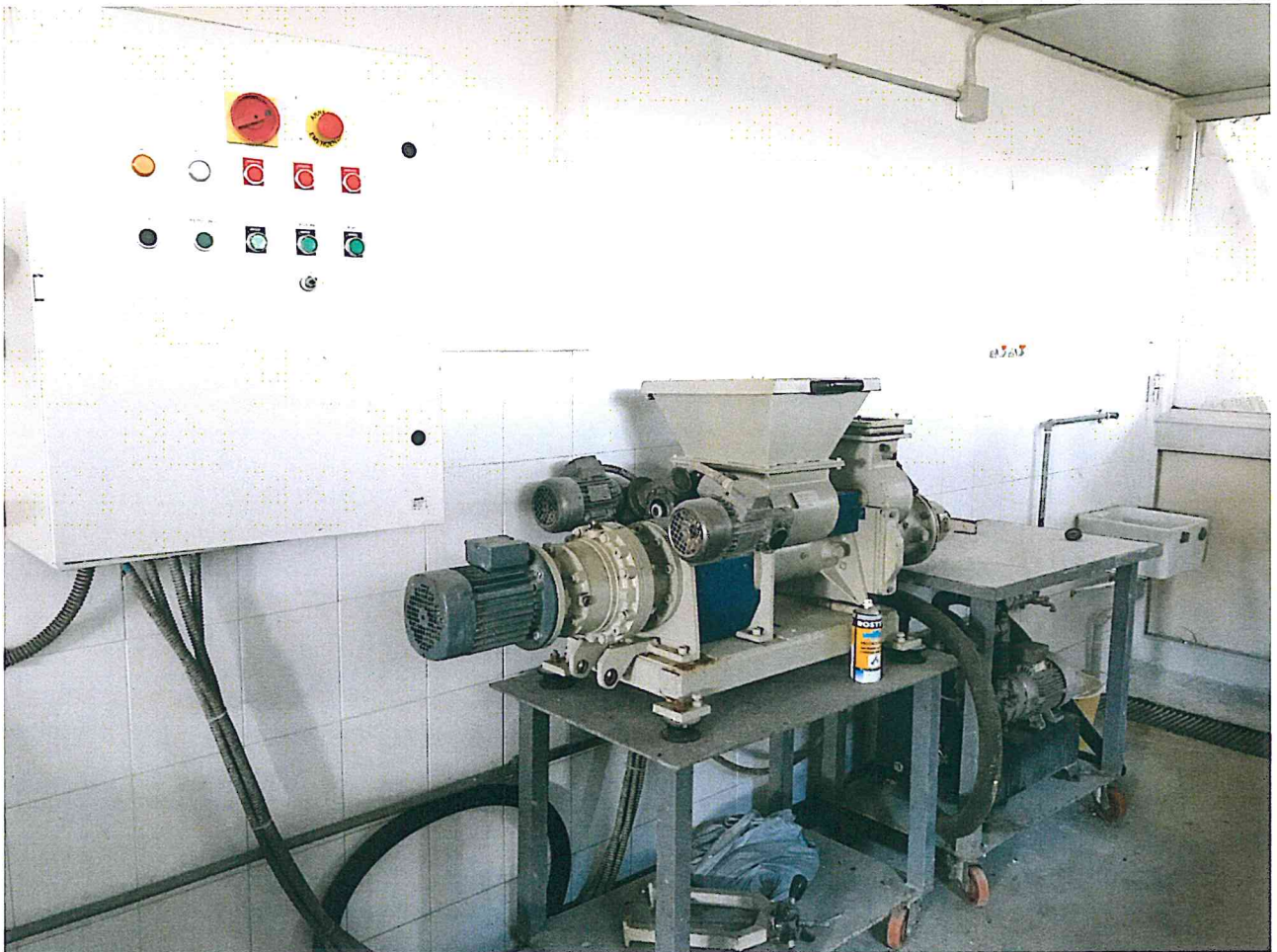
N38 MINIESTRUSORE
